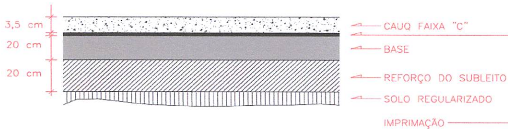
Figura 2.8 - Seção Tipo I
