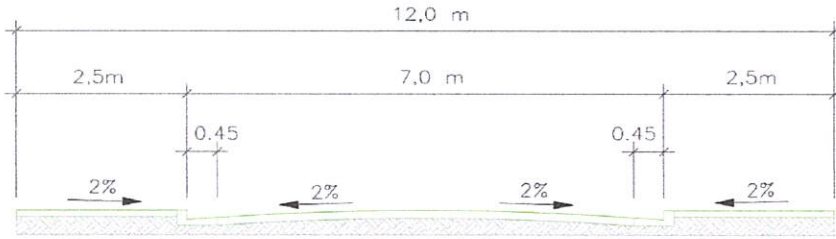
Figura 2.3 – Seção Tipo II
