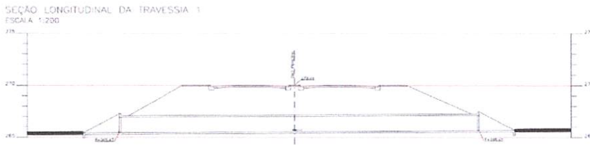
Figura 2.7 - Bueiro de Travessia Acesso Principal
