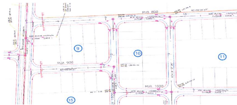
Figura 2.6 - Projeto de Drenagem - Detalhe Ampliado
