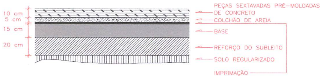
Figura 2.9 - Seção Tipo II
