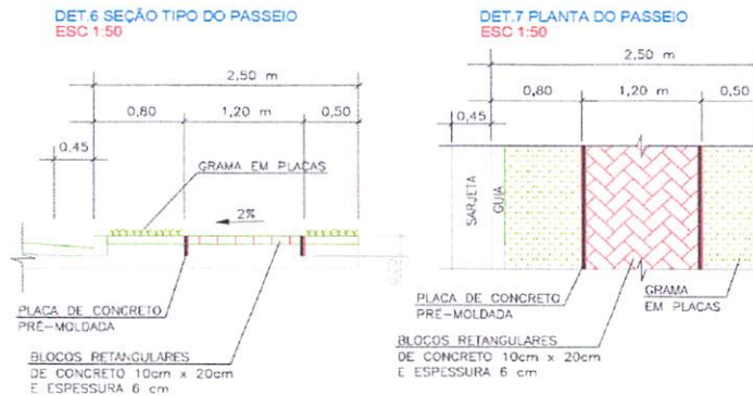
Figura 2.13 – Detalhes Passeio
