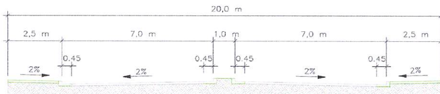
Figura 2.2 – Seção Tipo I
